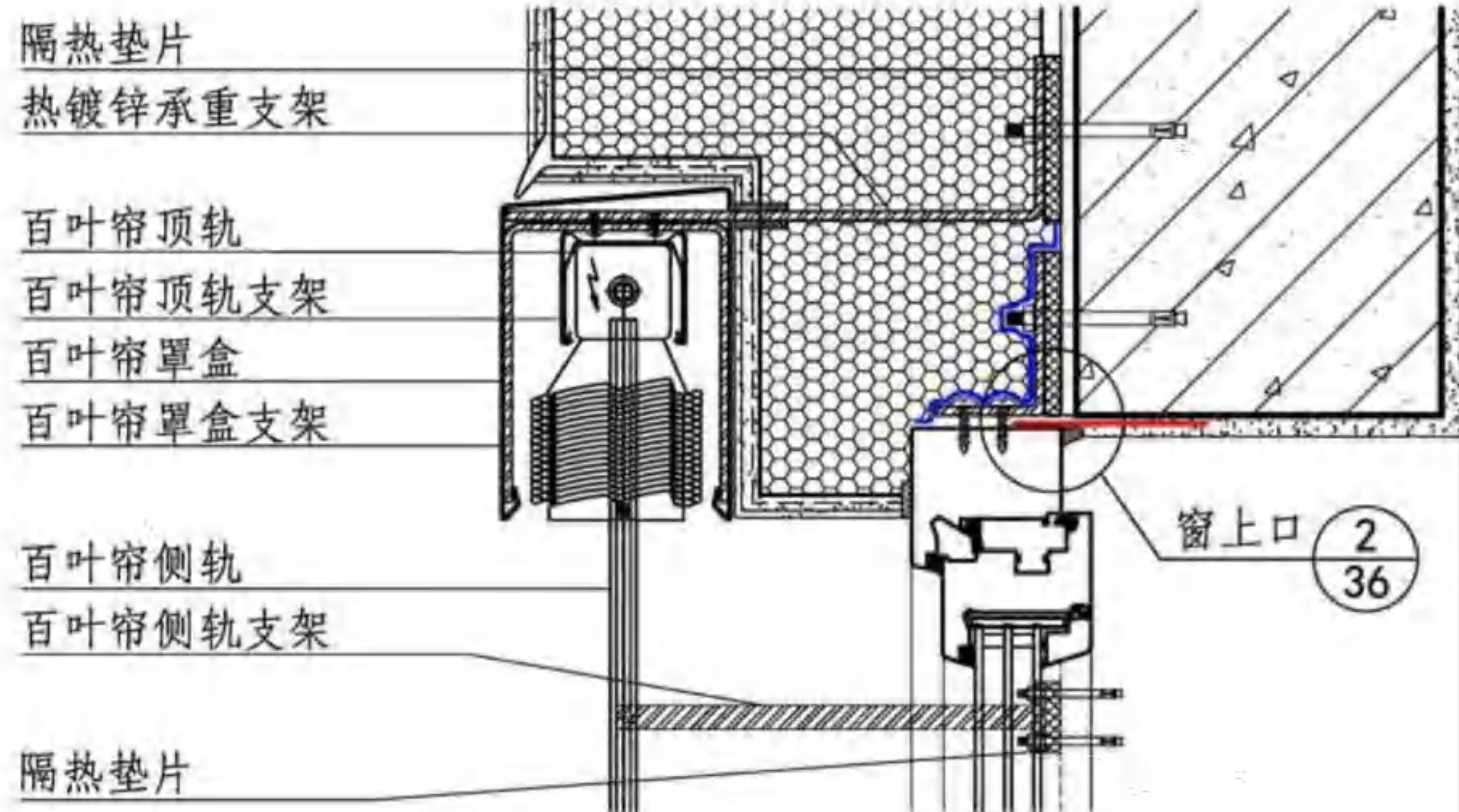
① 嵌装式Z型铝合金百叶帘上口一
