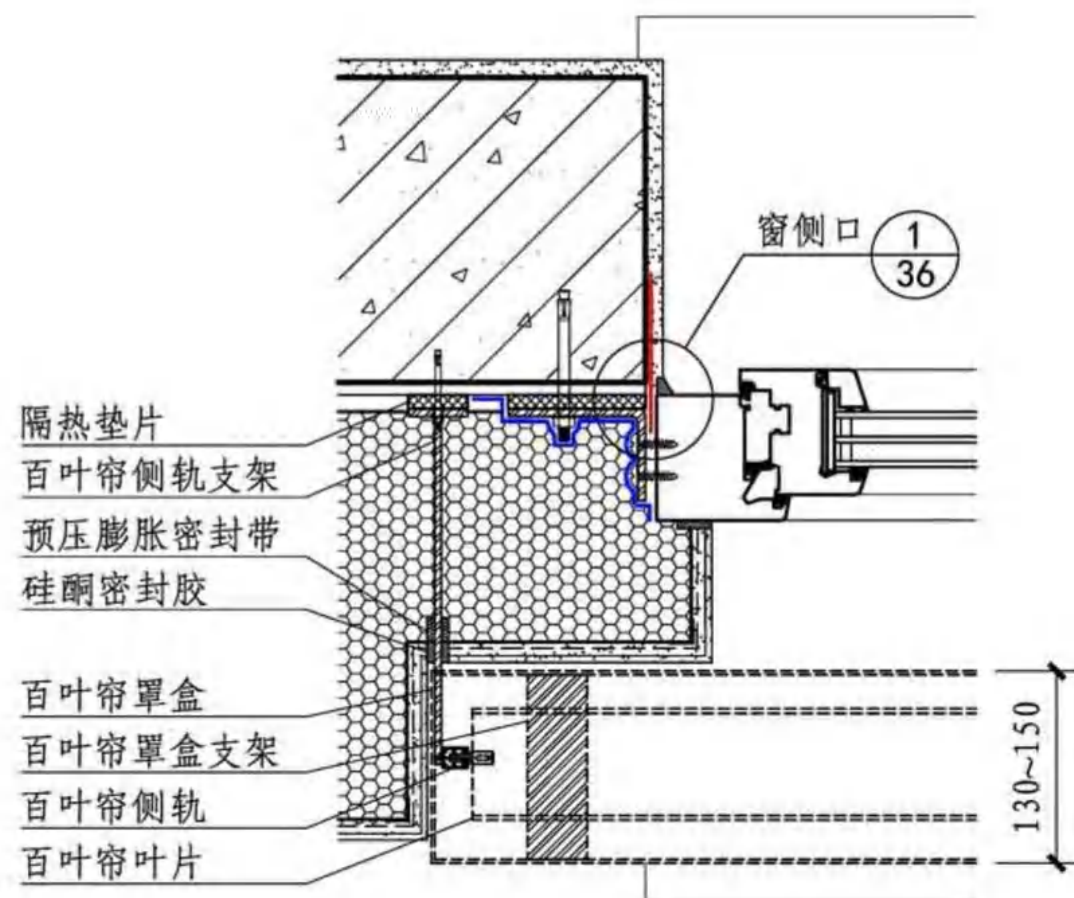
③ 嵌装式Z型铝合金百叶帘侧口
