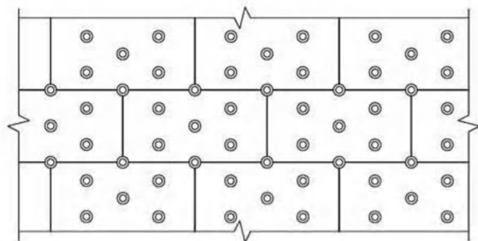
模塑聚苯板、岩棉板锚栓布局图
