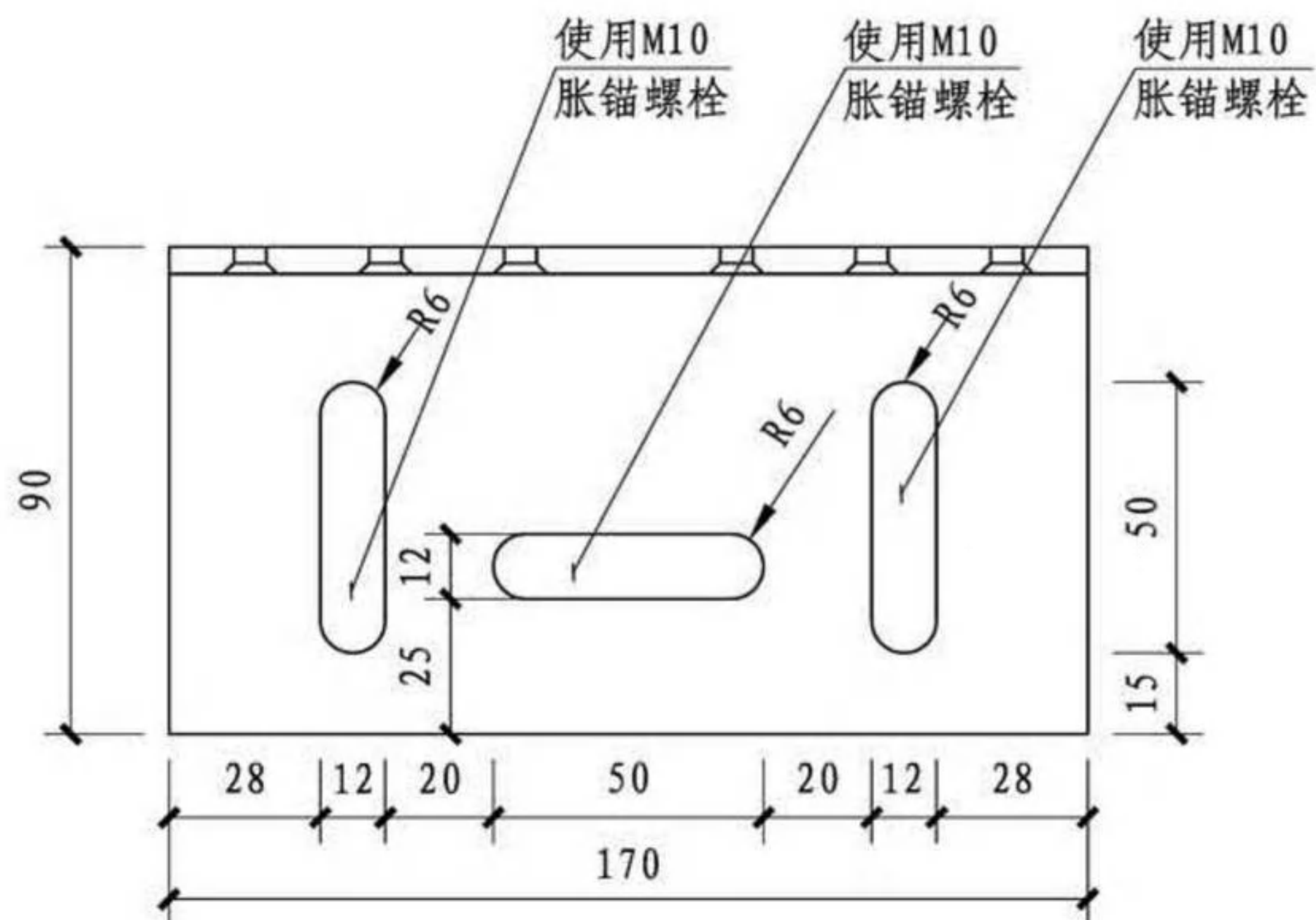
前视图
