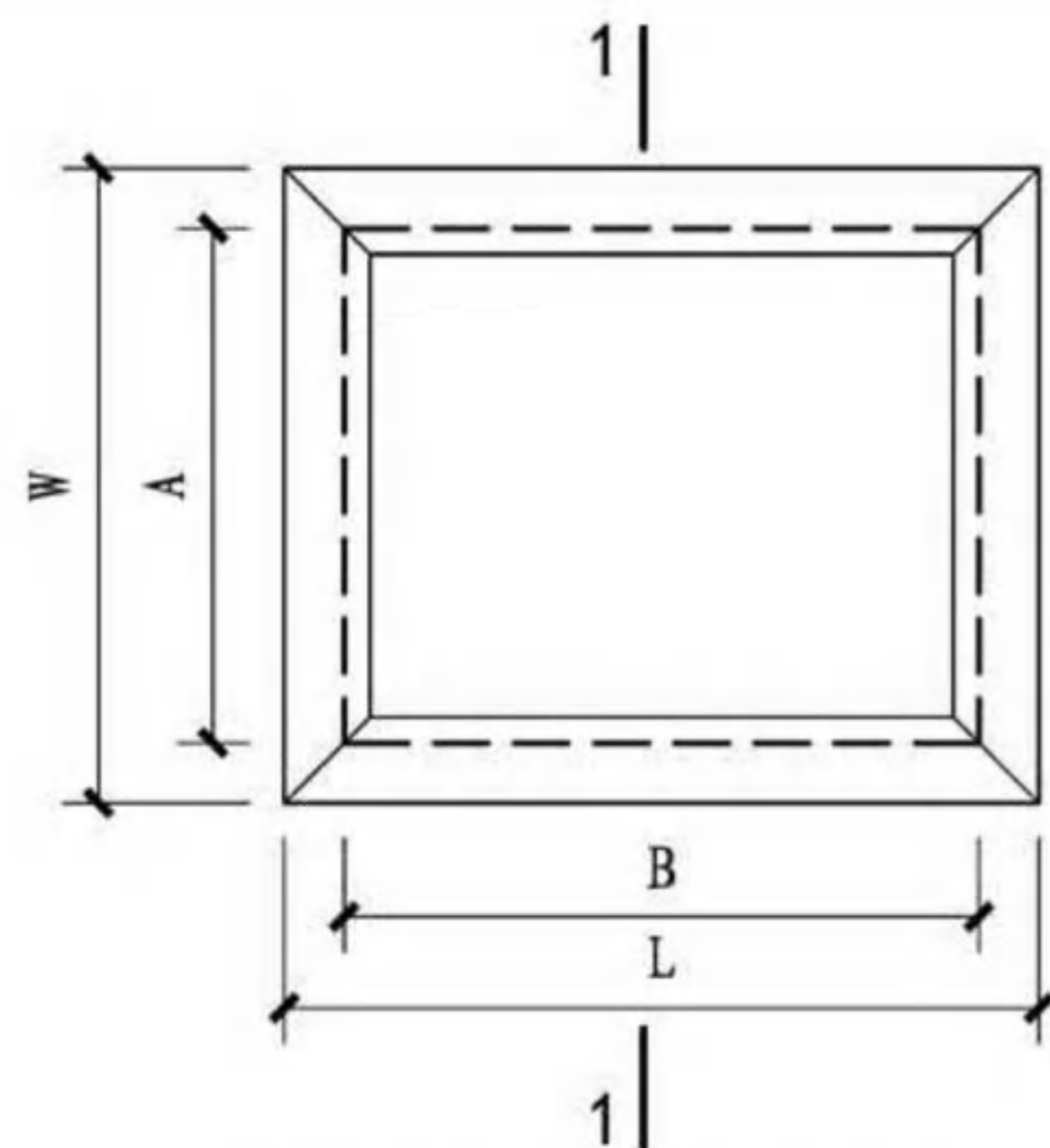
平屋顶天窗平面尺寸图
