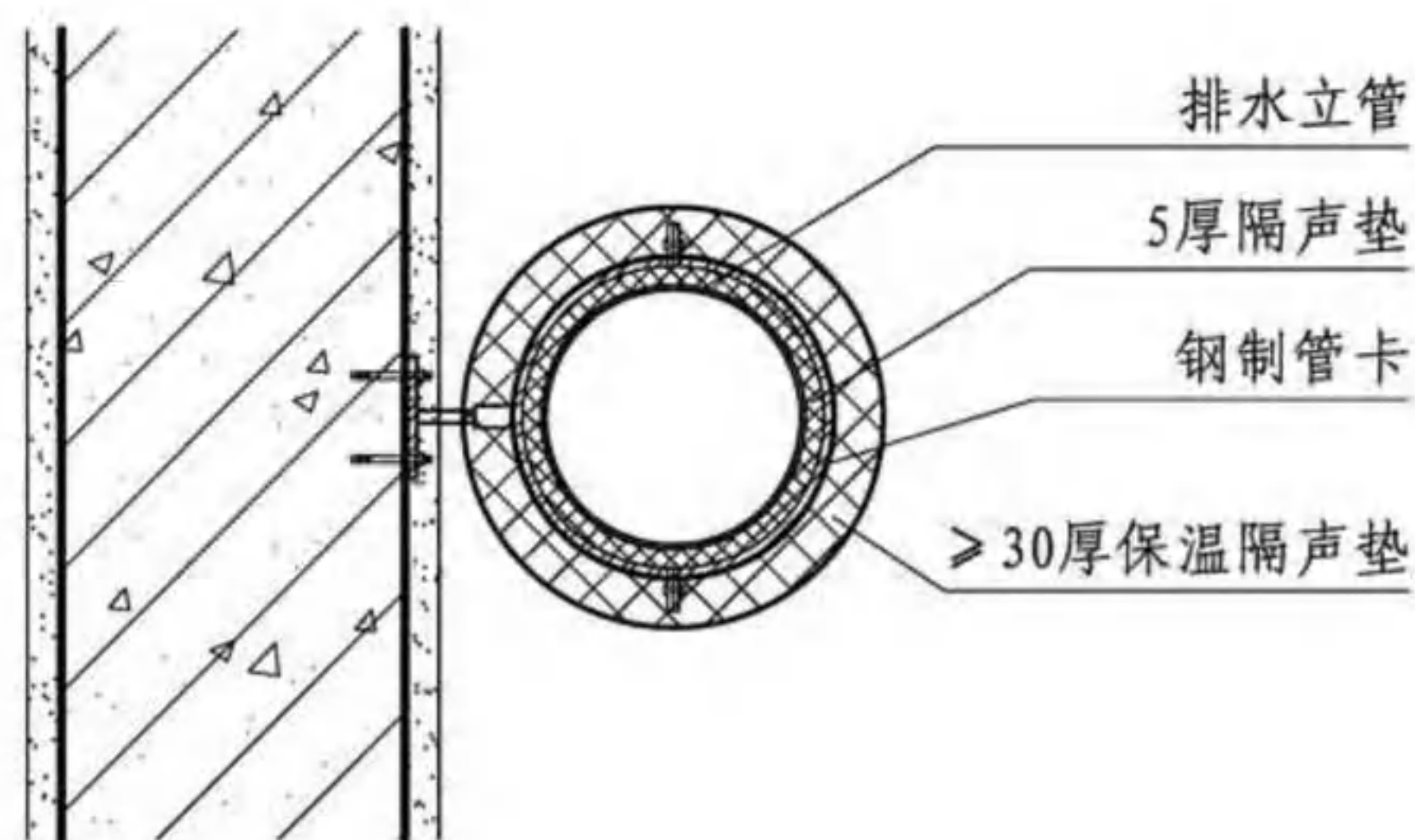
排水立管
