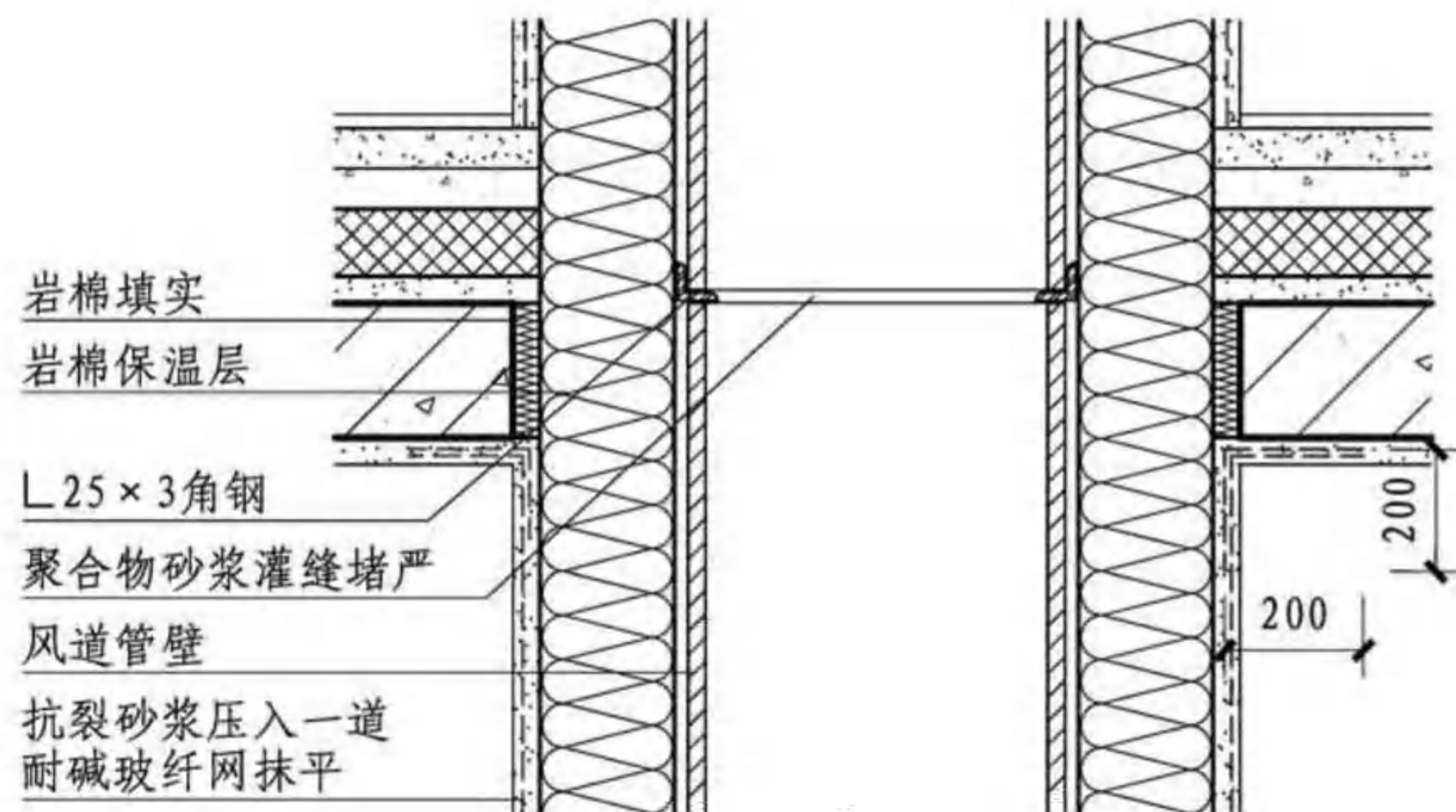
室内穿楼板风道
