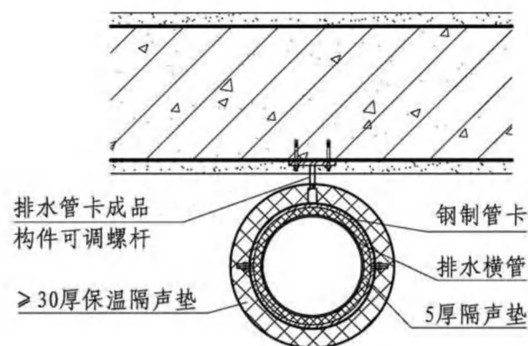
排水横管
