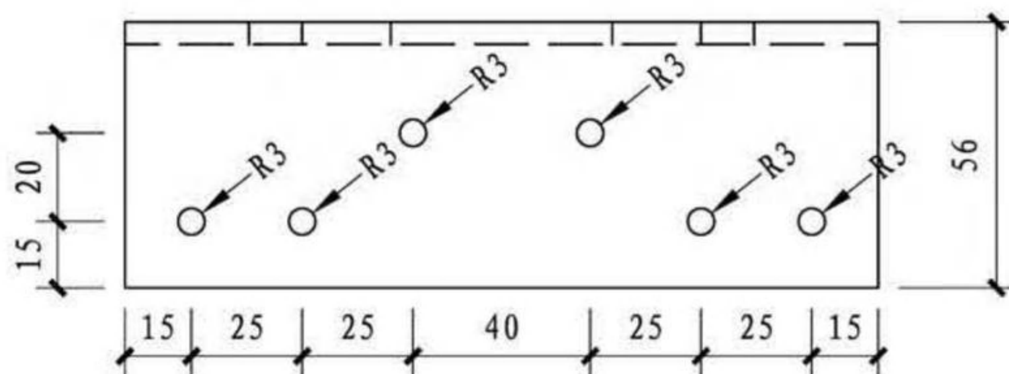
俯视图
