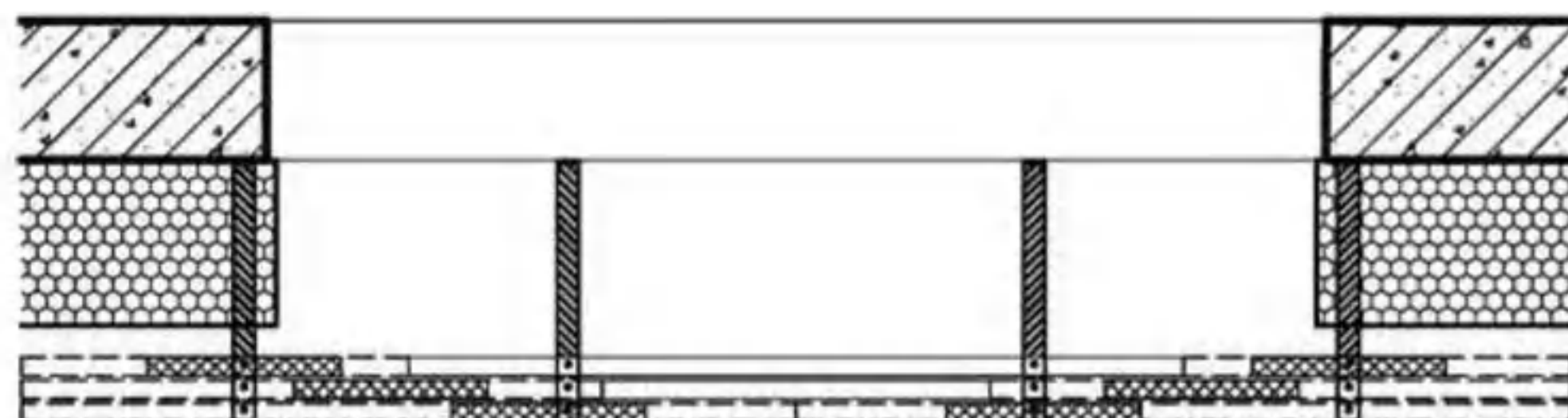
外挂推拉滑动式百叶窗开启、关闭状态示意图
