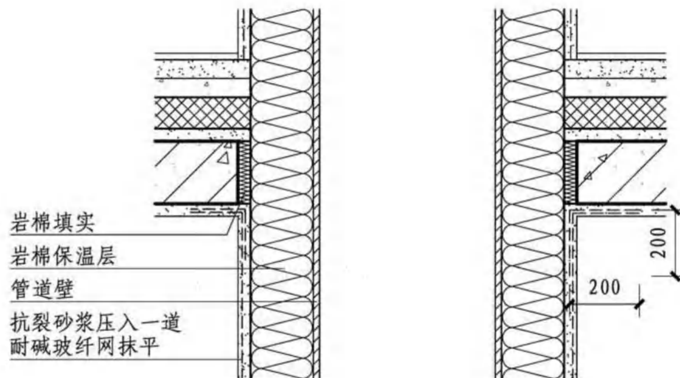
室内穿楼板管道
