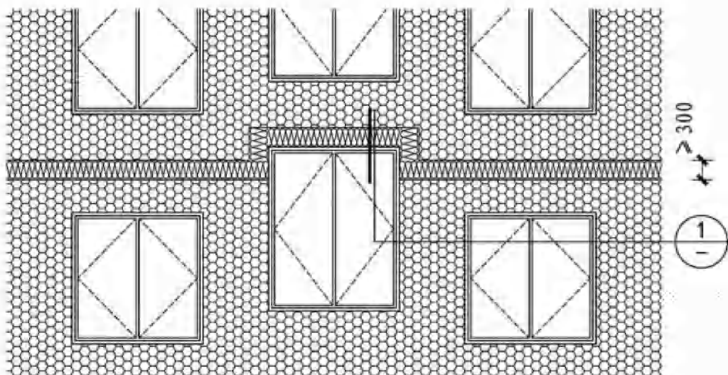
防火隔离带设置 (窗口上移)
