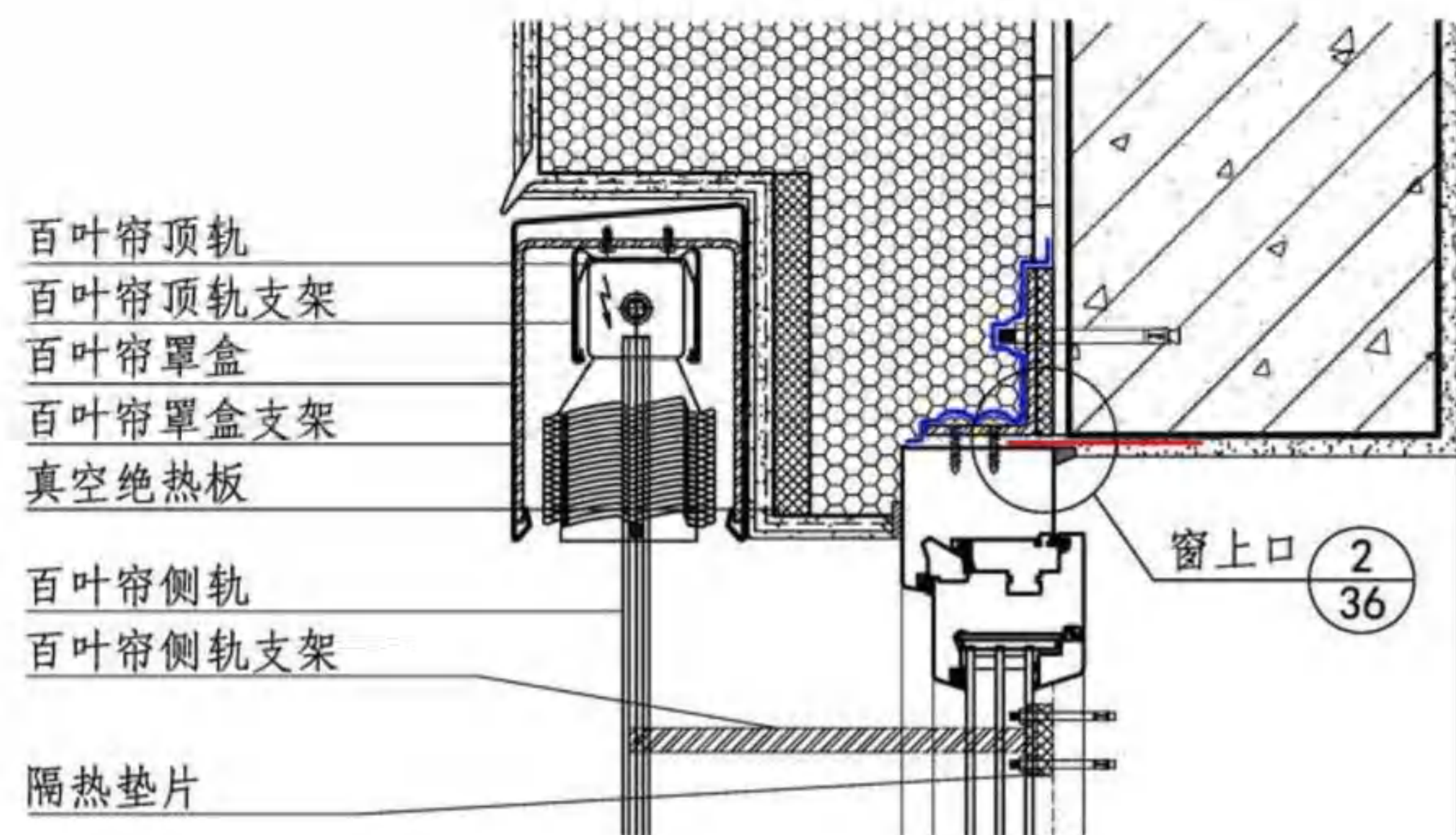
② 嵌装式Z型铝合金百叶帘上口二
