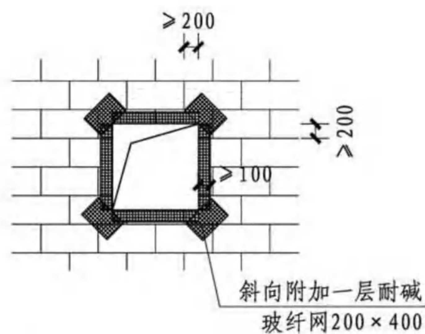
门窗洞口耐碱玻纤网铺设示意图
