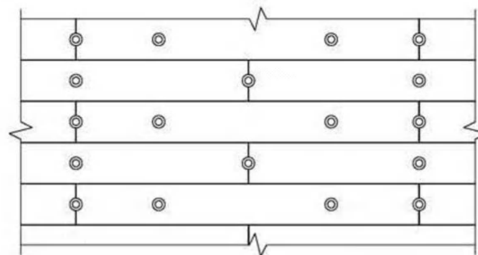
岩棉条锚栓布局图
