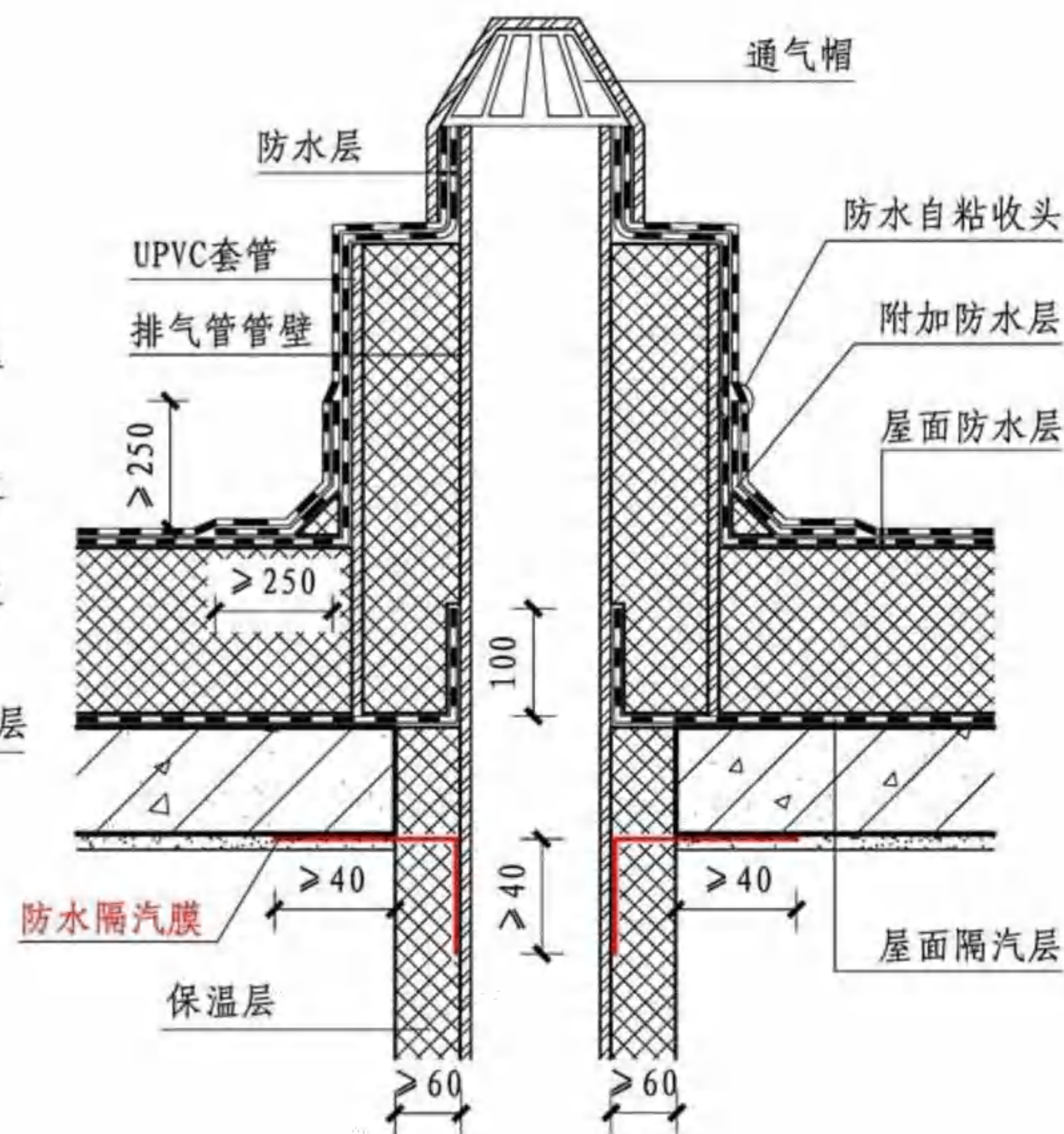
排气管出屋面
