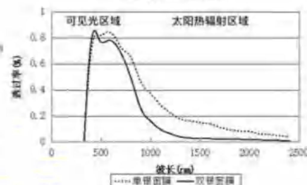
隔热窗膜节能示意图
